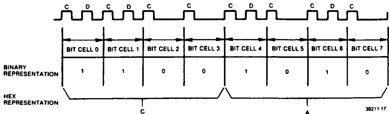
FIGURE 4-1. BYTE
